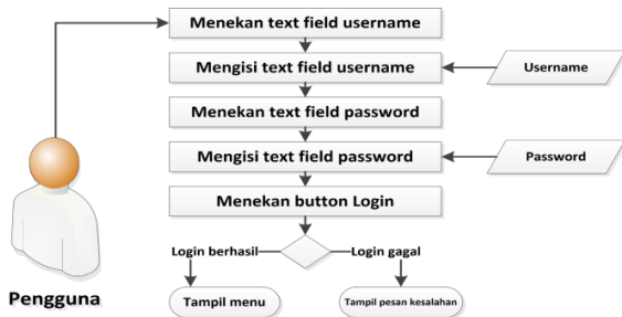
Gambar 4 Alur seorang user saat mengakses fitur Login pada aplikasi
