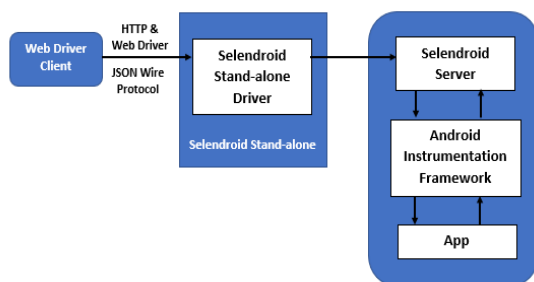
Gambar 1 Arsitektur Selendroid
