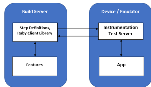
Gambar 2 Arsitektur Calabash
