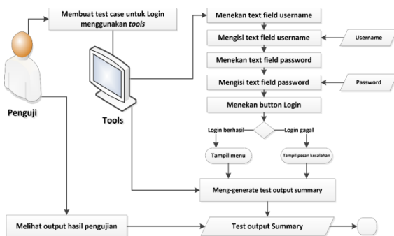
Gambar 5 Alur pengujian fitur login menggunakan alat pengujian
